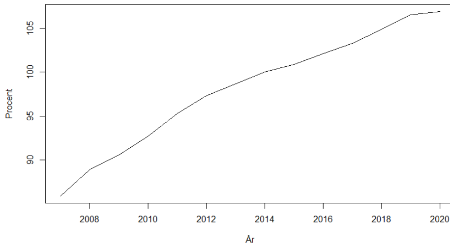
Figur 5: Törnqvist prisindeks, 2014=100.
